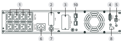
Вид сзади: ИБП ИМПУЛЬС ФРИСТАЙЛ 1500 ВА
