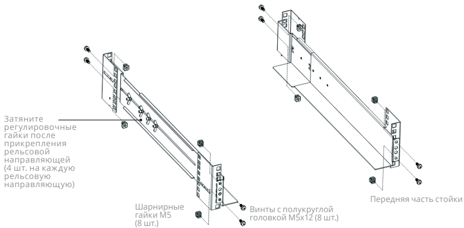
Рисунок 2. Крепление направляющих
