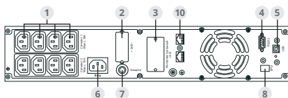
Вид сзади: ИБП ИМПУЛЬС ФРИСТАЙЛ 1000 ВА
