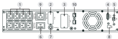
Вид сзади: ИБП ИМПУЛЬС ФРИСТАЙЛ 3000 ВА
