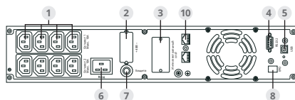
Вид сзади: ИБП ИМПУЛЬС ФРИСТАЙЛ 2000 ВА
